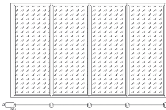
Verrière, Profils carrés, montants intermédiaires assemblés en tenon/mortaise
