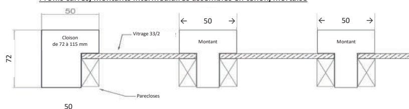
Verrière, Profils carrés, petits bois intermédiaires rapportés/collés
